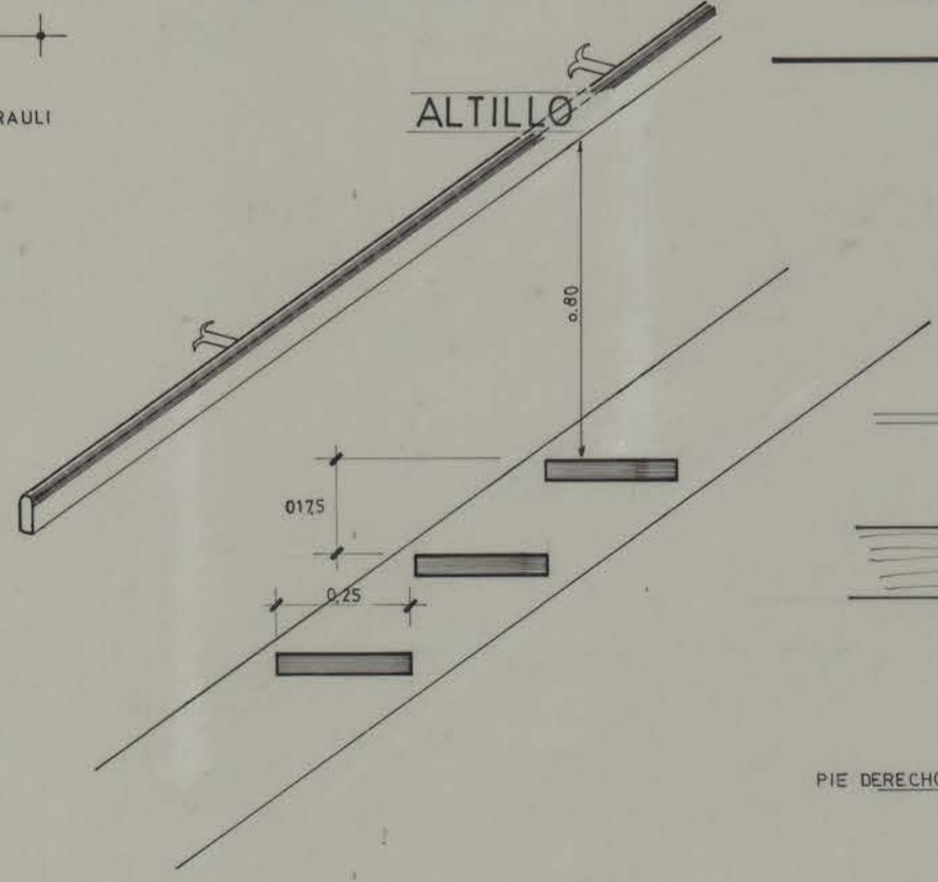
DET. GRADAS ESC. 1:10
