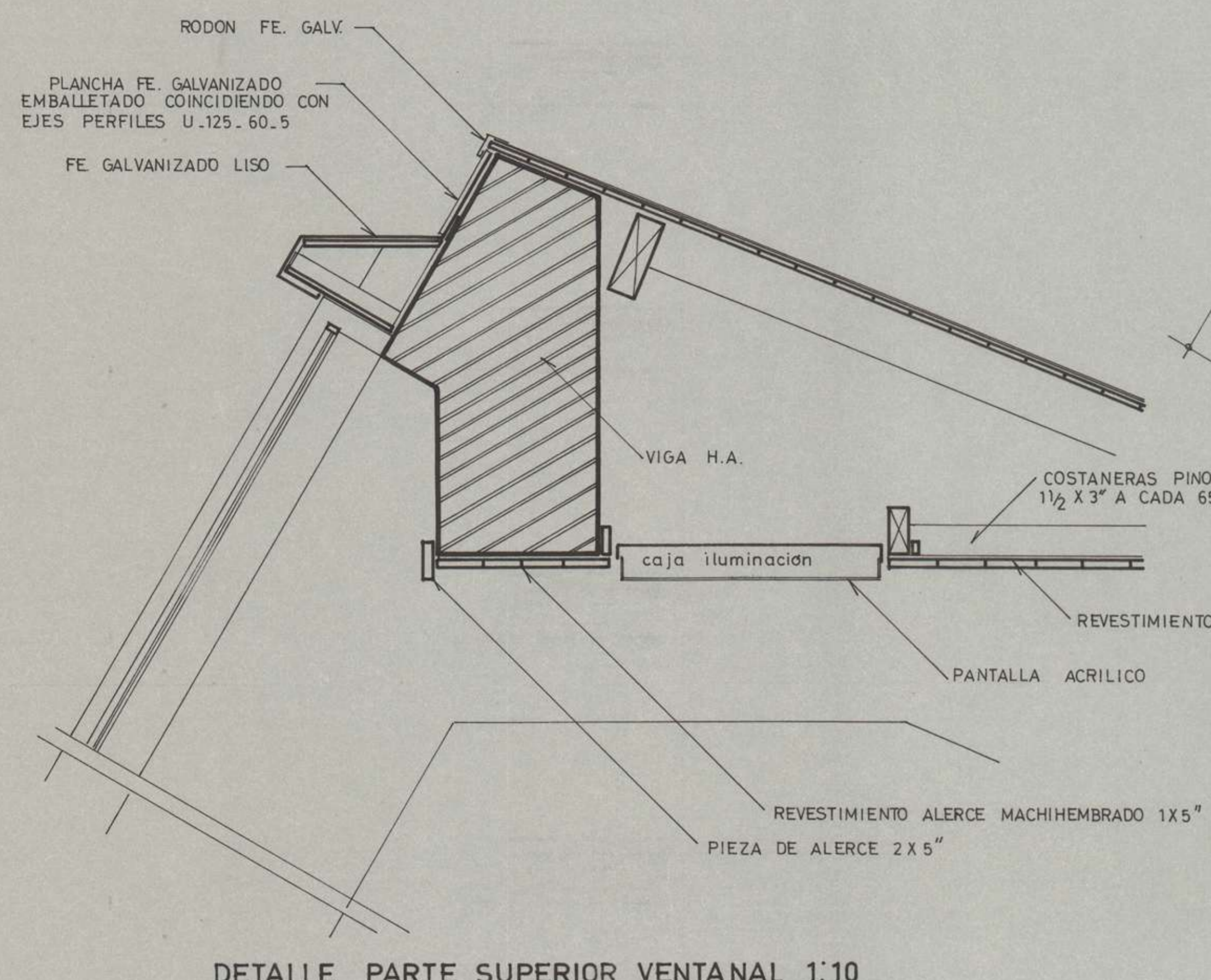
DETALLE PARTE SUPERIOR VENTANAL 1:10
