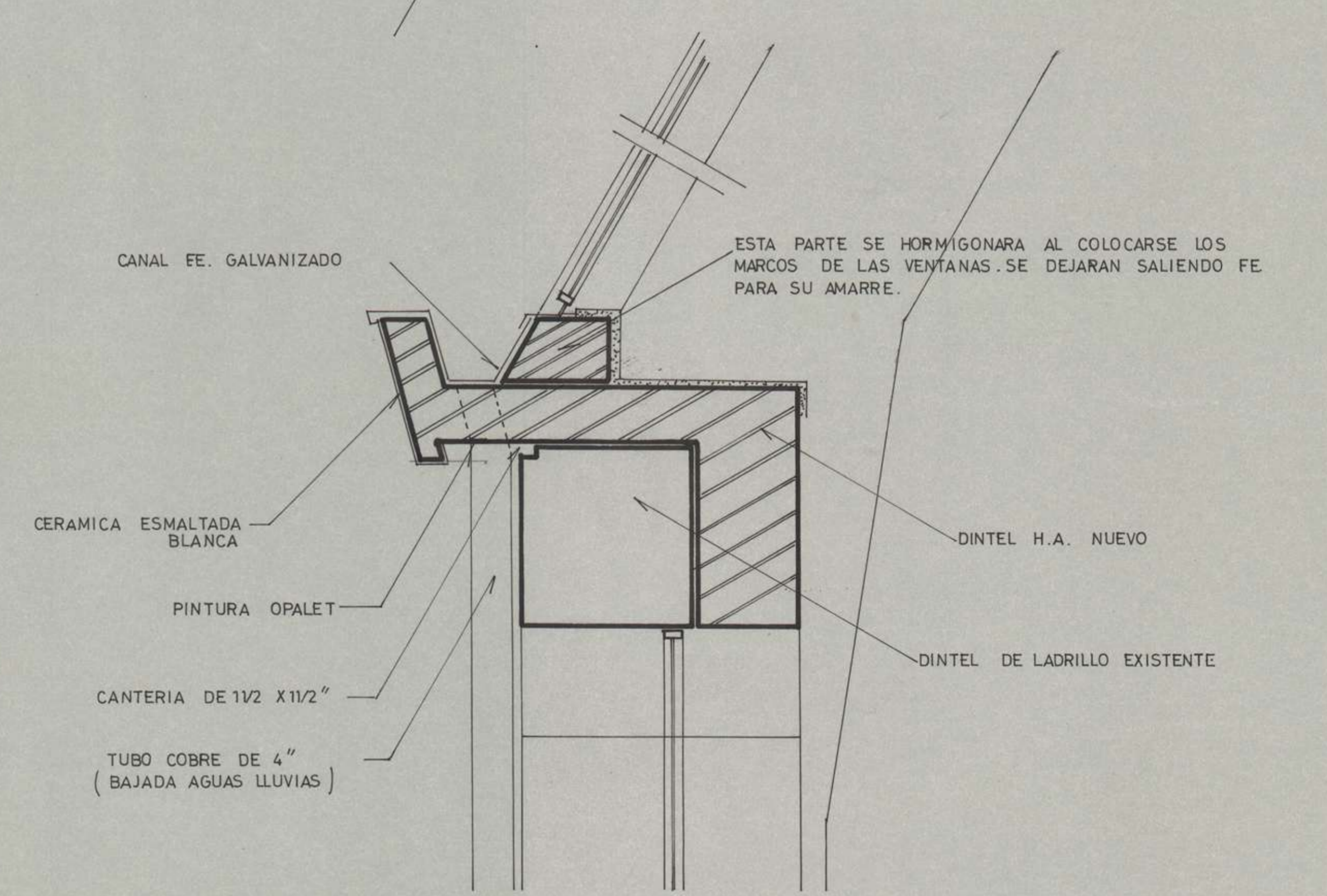
DETALLE PARTE INFERIOR DEL VENTANAL 1:10
