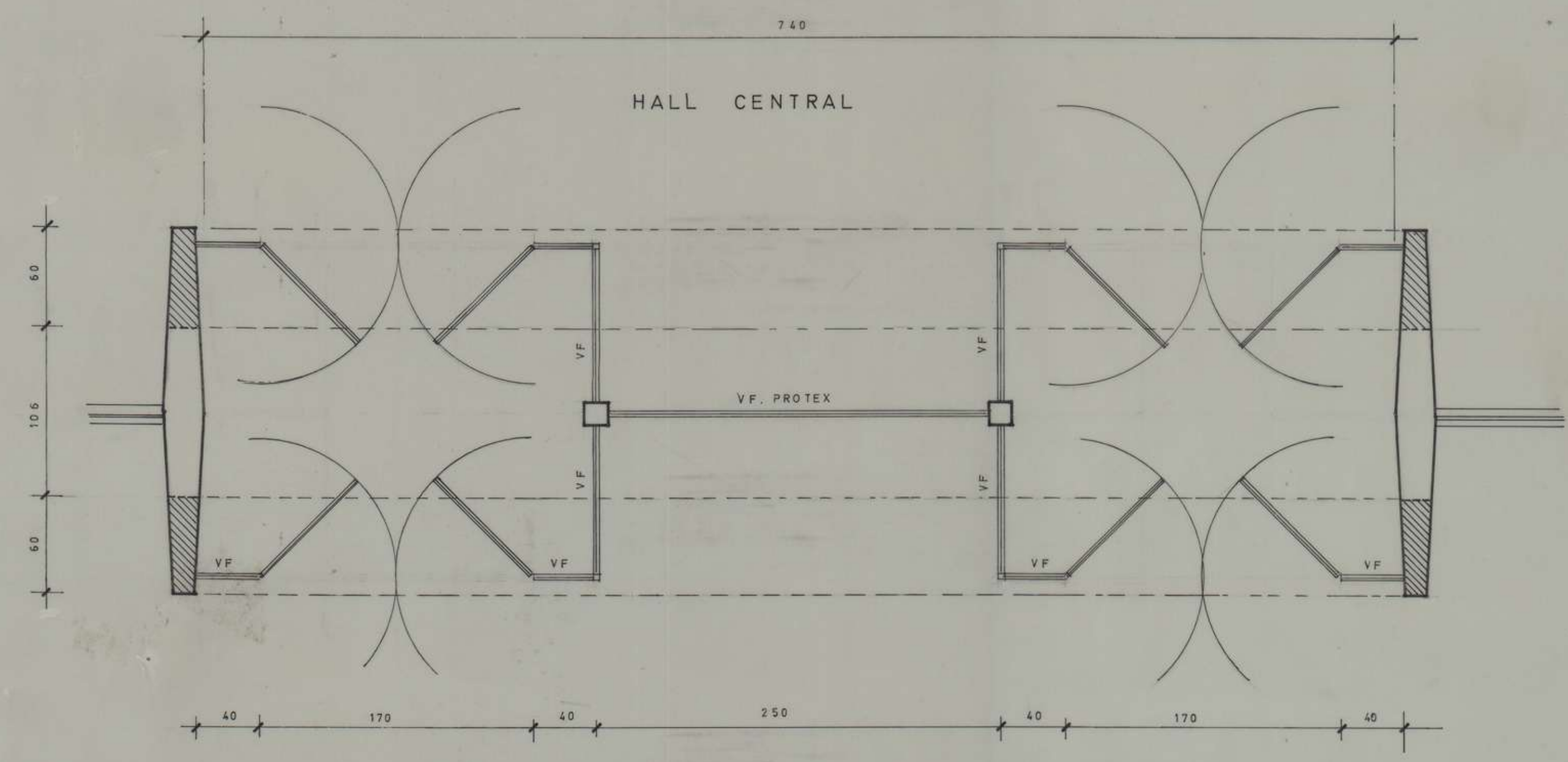
PLANTA ESC. 1:25
