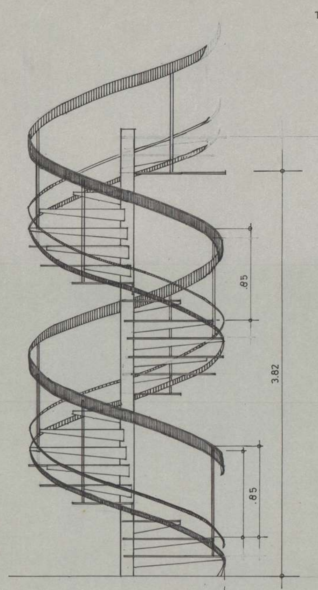
ALZADO 1:20
