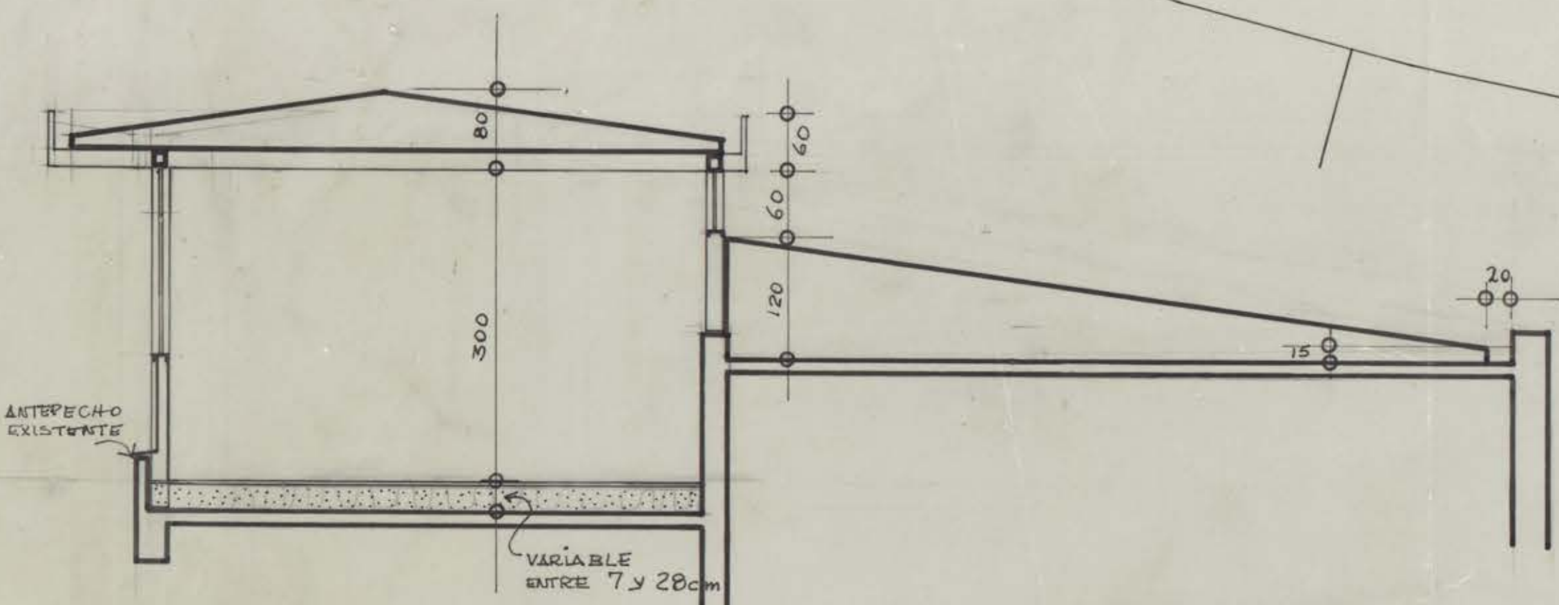
CORTE A
