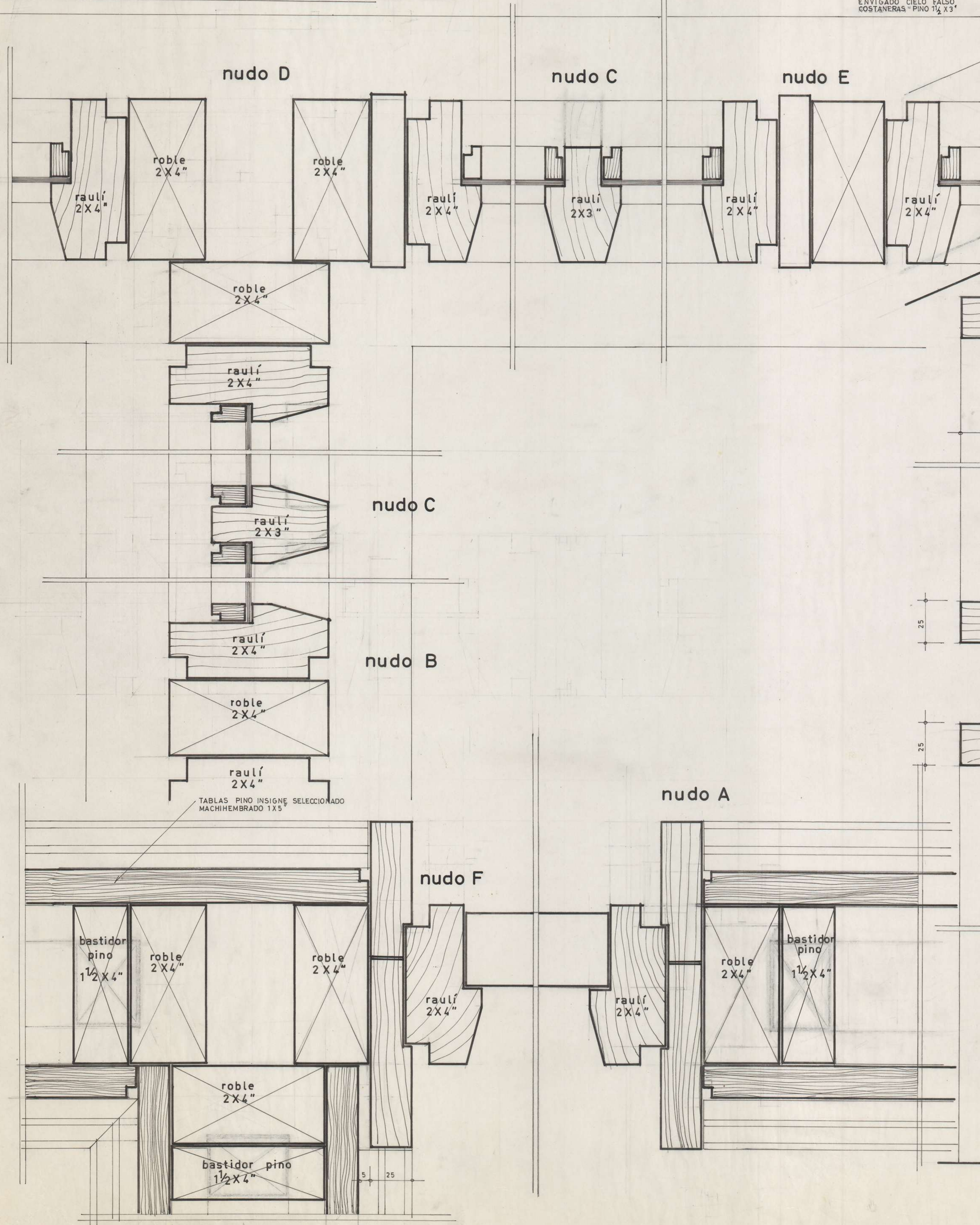
ESTRUCTURA TABIQUES 1:20
