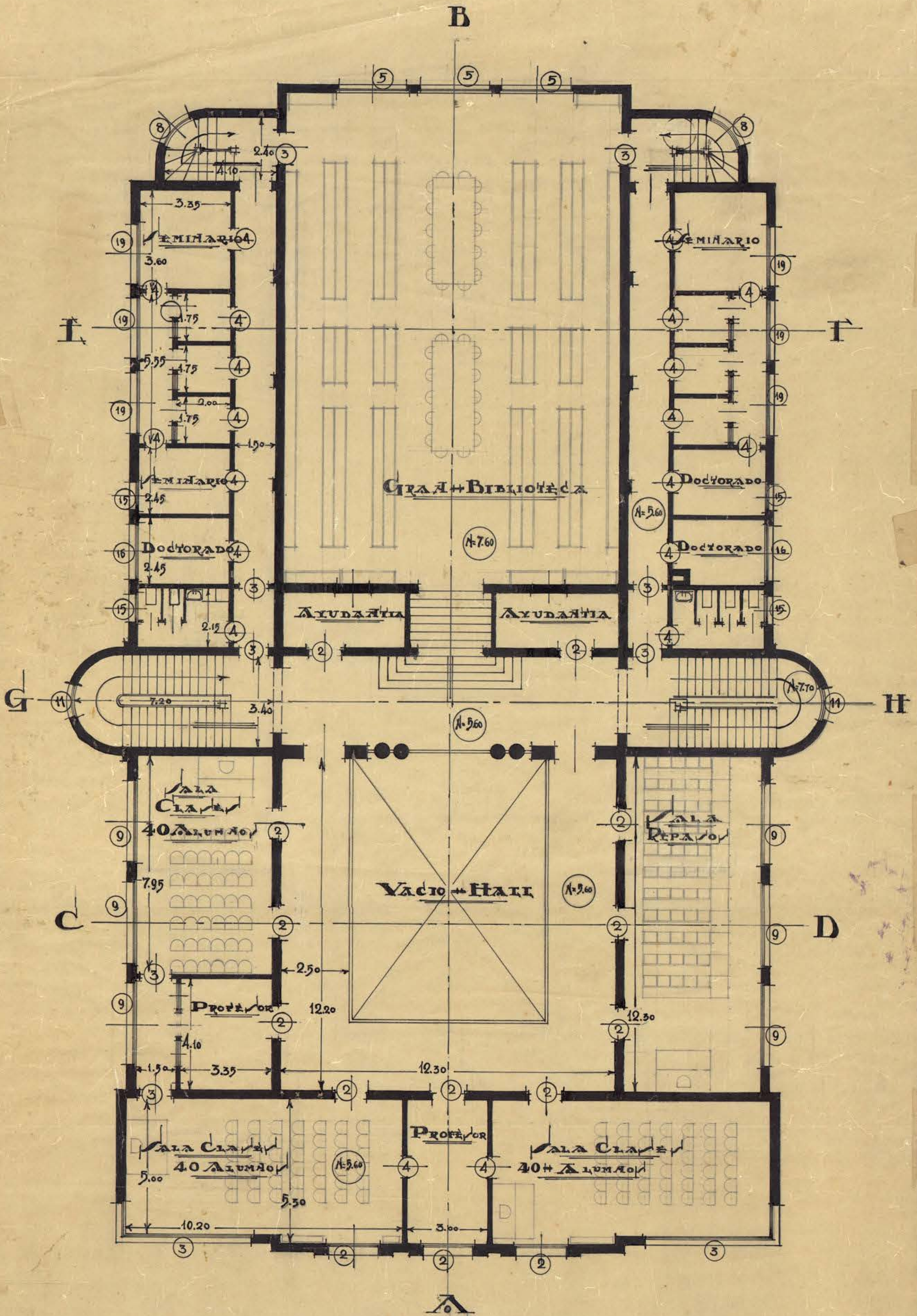
PLANO DEL SEGUNDO PISO
