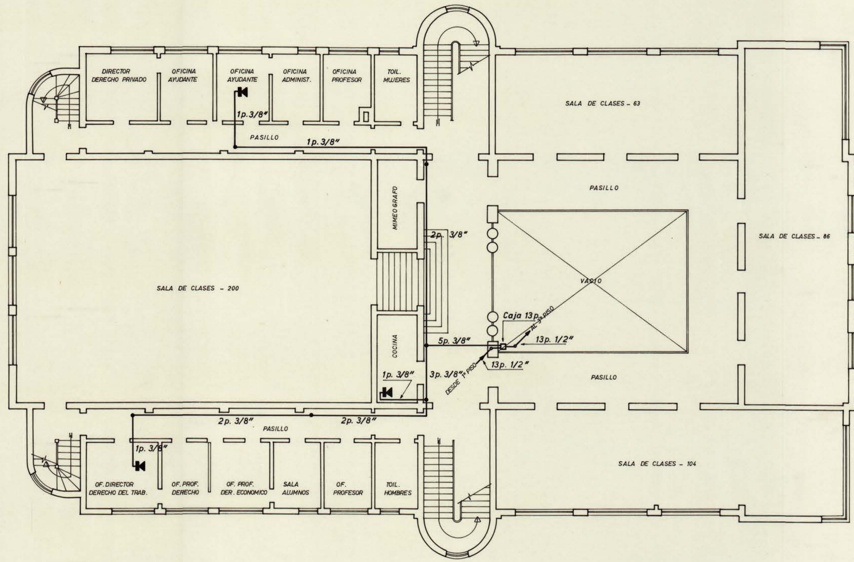
PLANTA DEL SEGUNDO PISO ESC. 1:100
