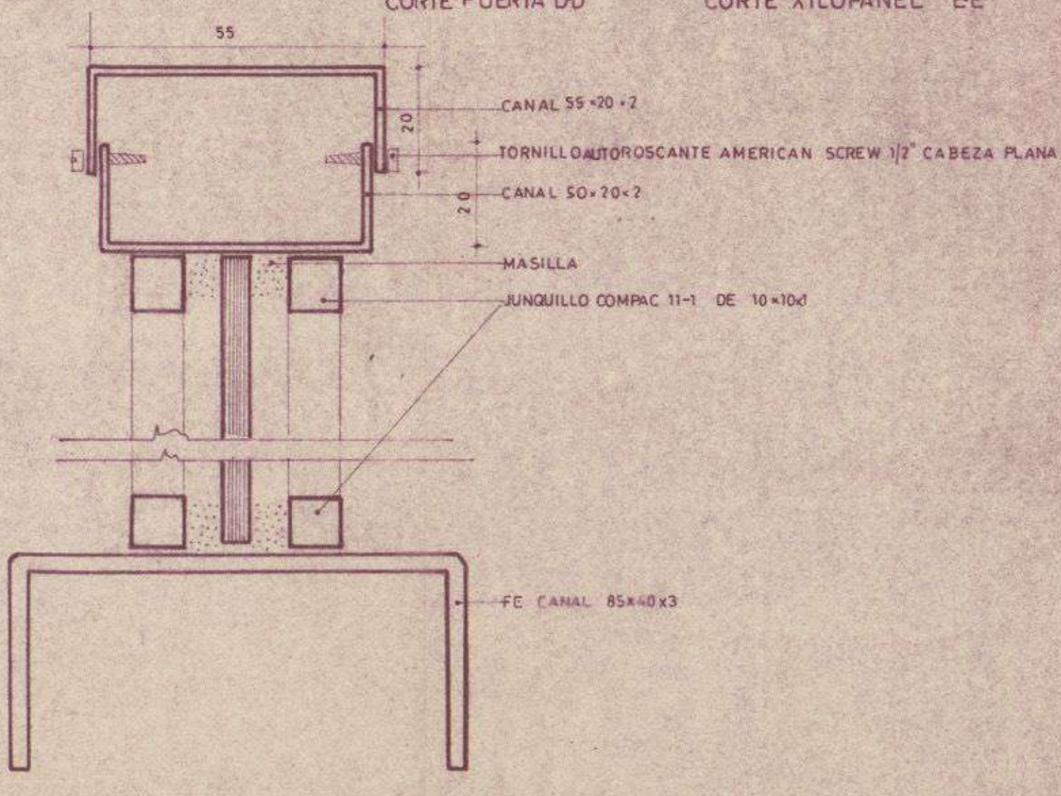
CORTE PUERTA DD CORTE XILOPANEL EE CORTE PANEL VIDRIADO FF
