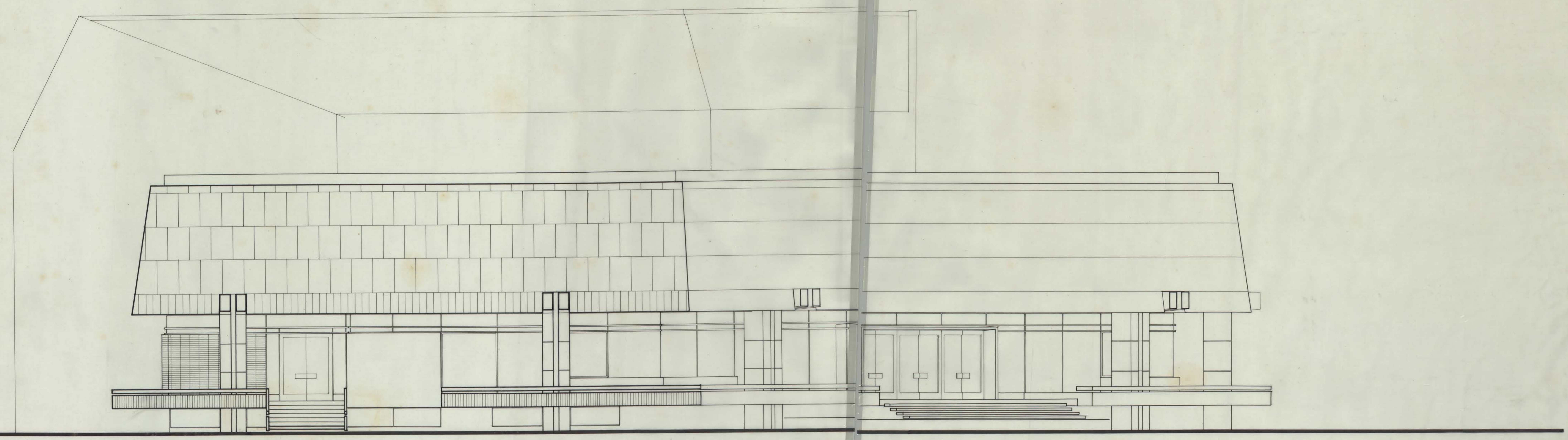
alzado norponiente (acceso escuela de arte)
