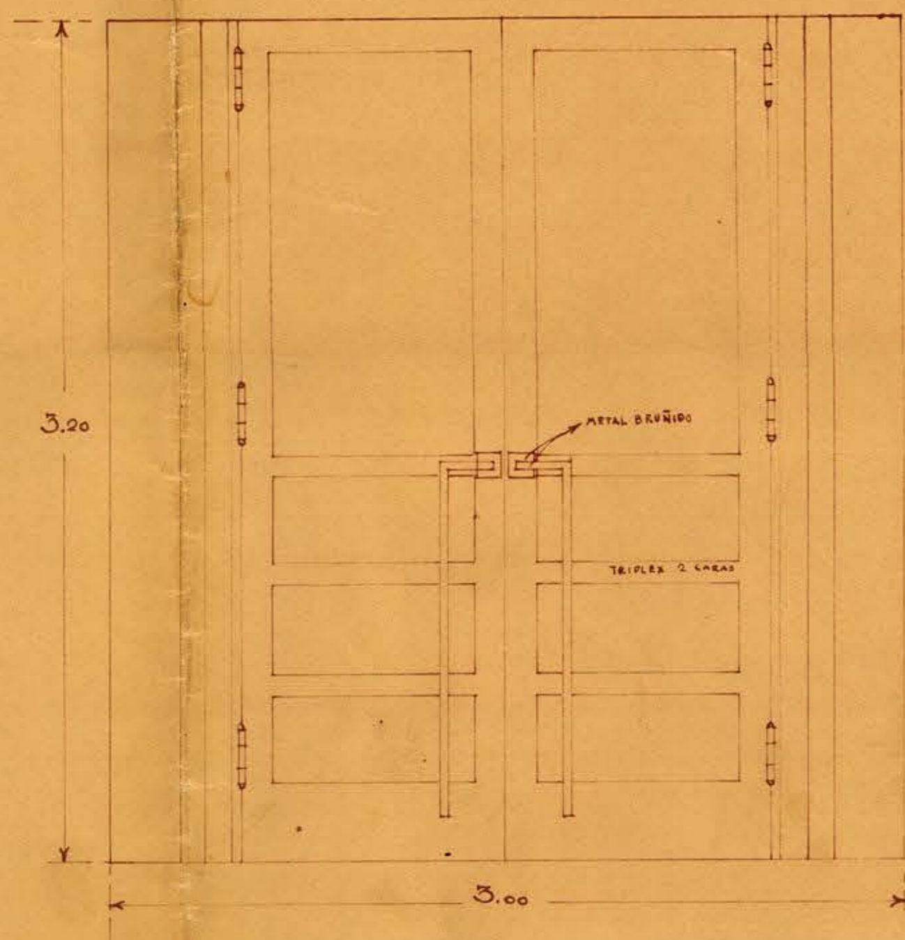
MAMPARA DE ENTRADA DATIENTES DE 3x5
