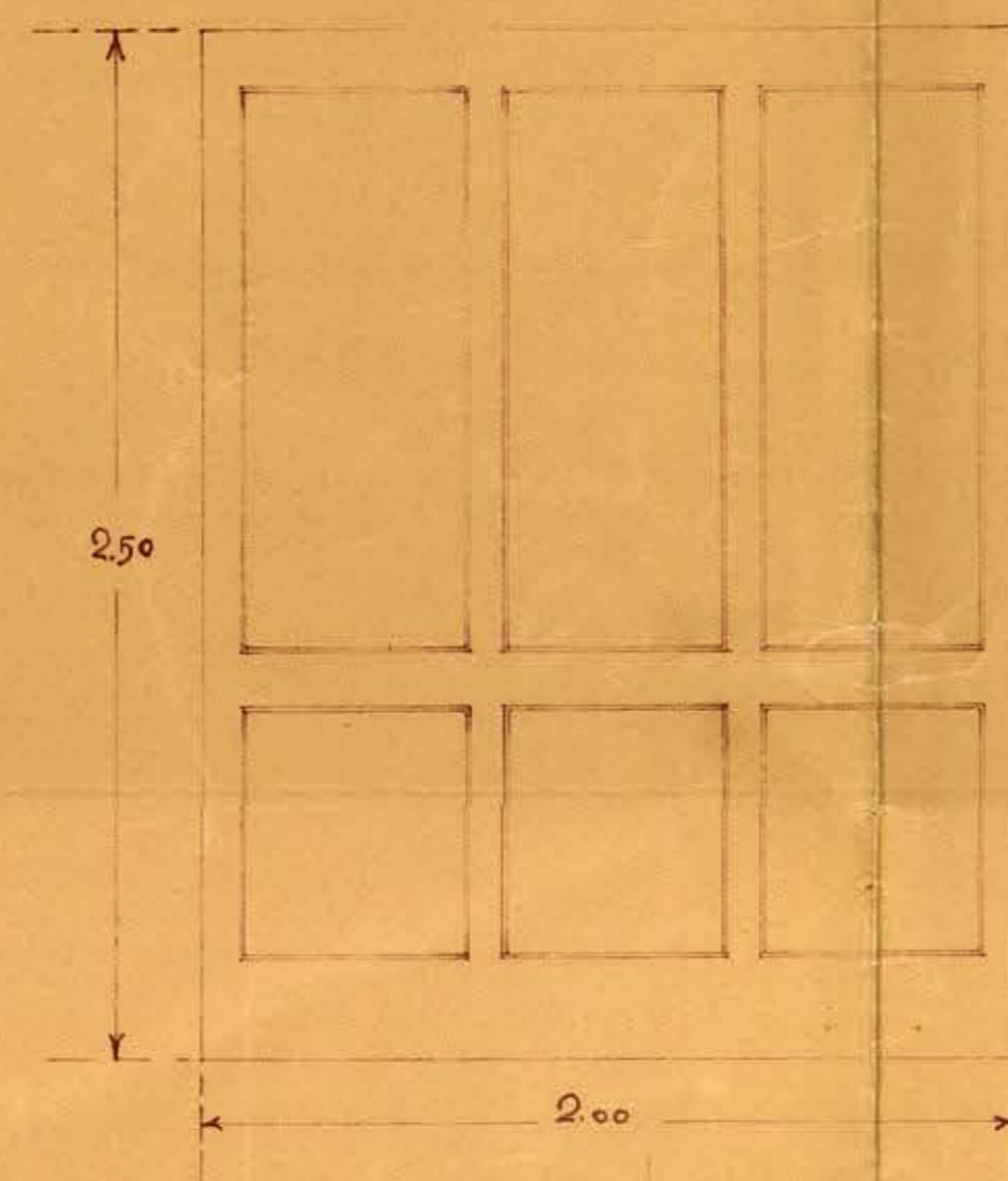
DIVISIONES DE LOS SEMINARIOS DATIENTES DE 2x4 MARCOS DE 3x4
