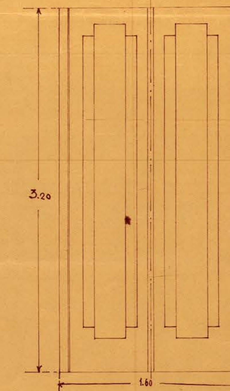
TIPO Nº 3 CANTIDAD 35 DATIENTES DE 2x4 MARCOS DE 3x4
