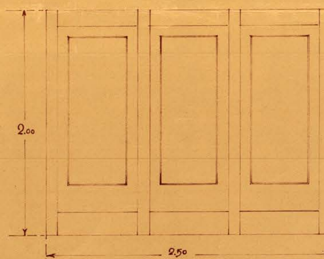
TIPO Nº 2 CANTIDAD 20 DATIENTES DE 2x4 MARCOS DE 3x4
