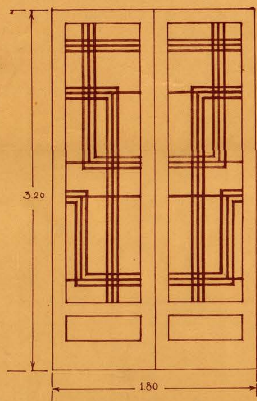
PUERTA REJA DE ENTRADA DATIENTES DE RAULI DE 3x5 MARCOS DE ROBLE DE 4x4
