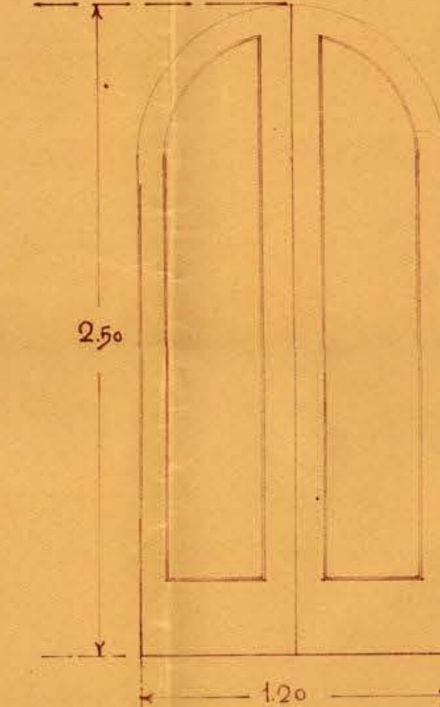
TIPO Nº 1 CANTIDAD 10 DATIENTES DE 2x4 MARCOS DE 3x4
