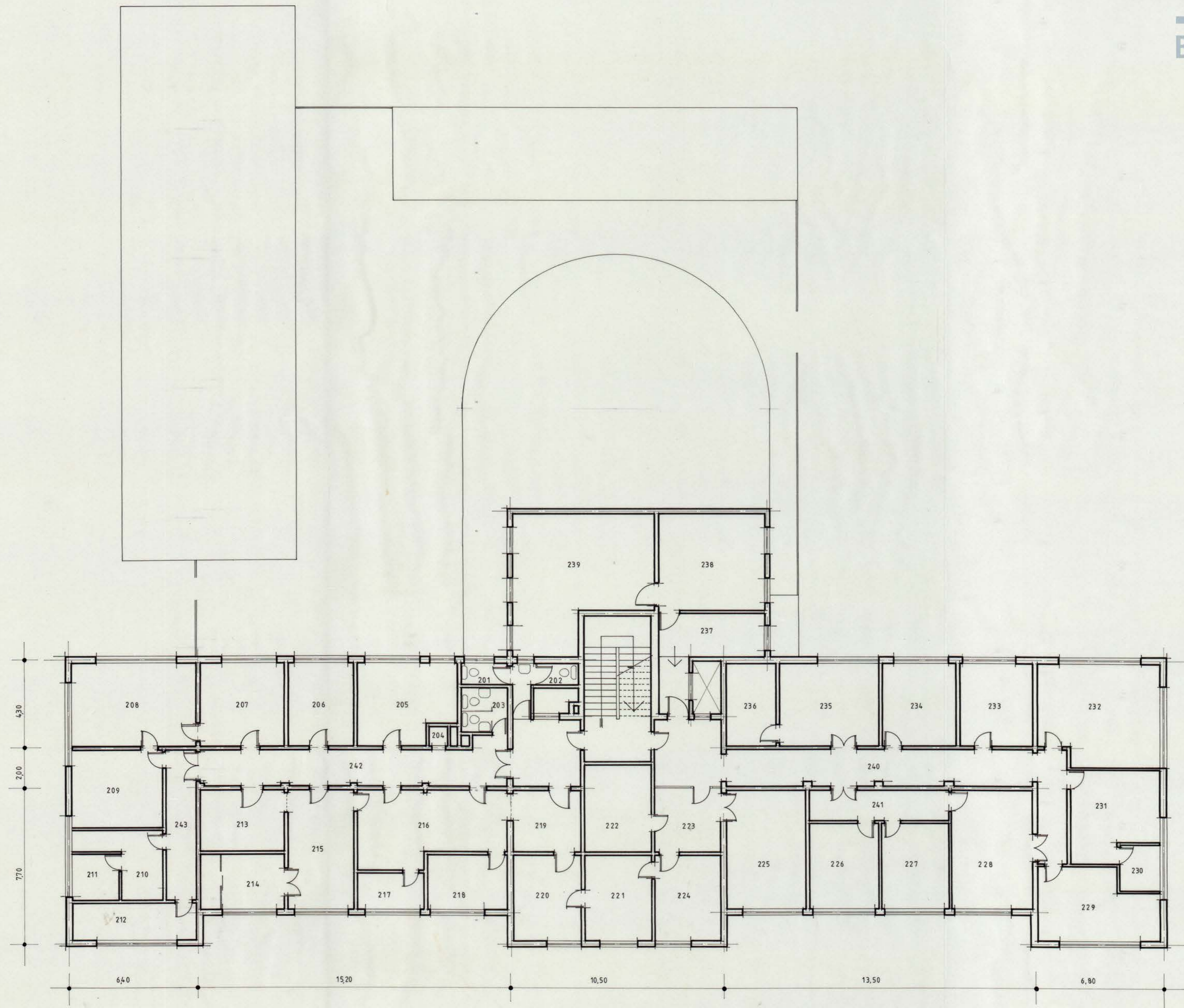
PLANTA 2do PISO EDIFICIO DE BIOLOGIA
