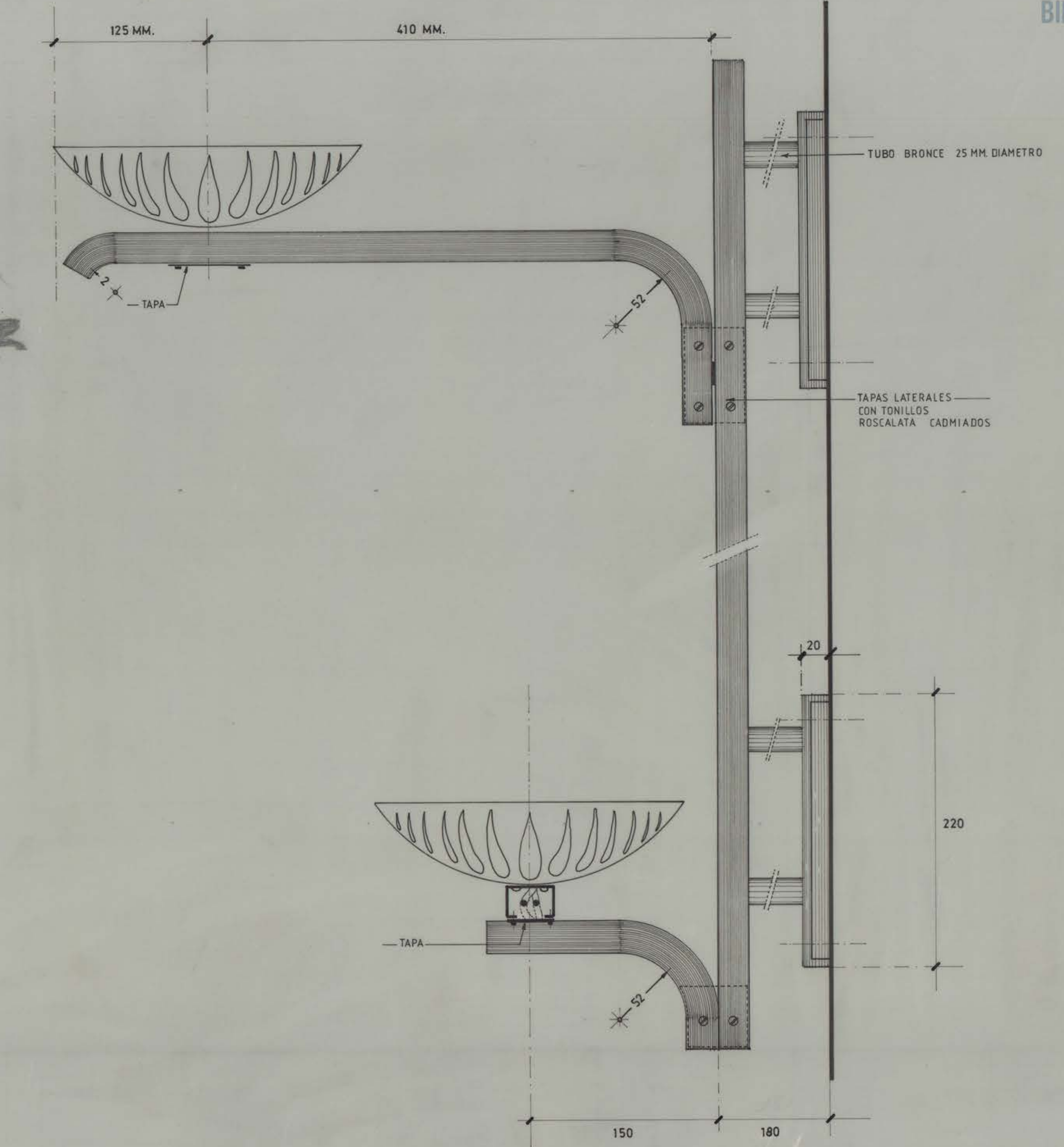
ELEVACION LATERAL ESC. 1:2,5
