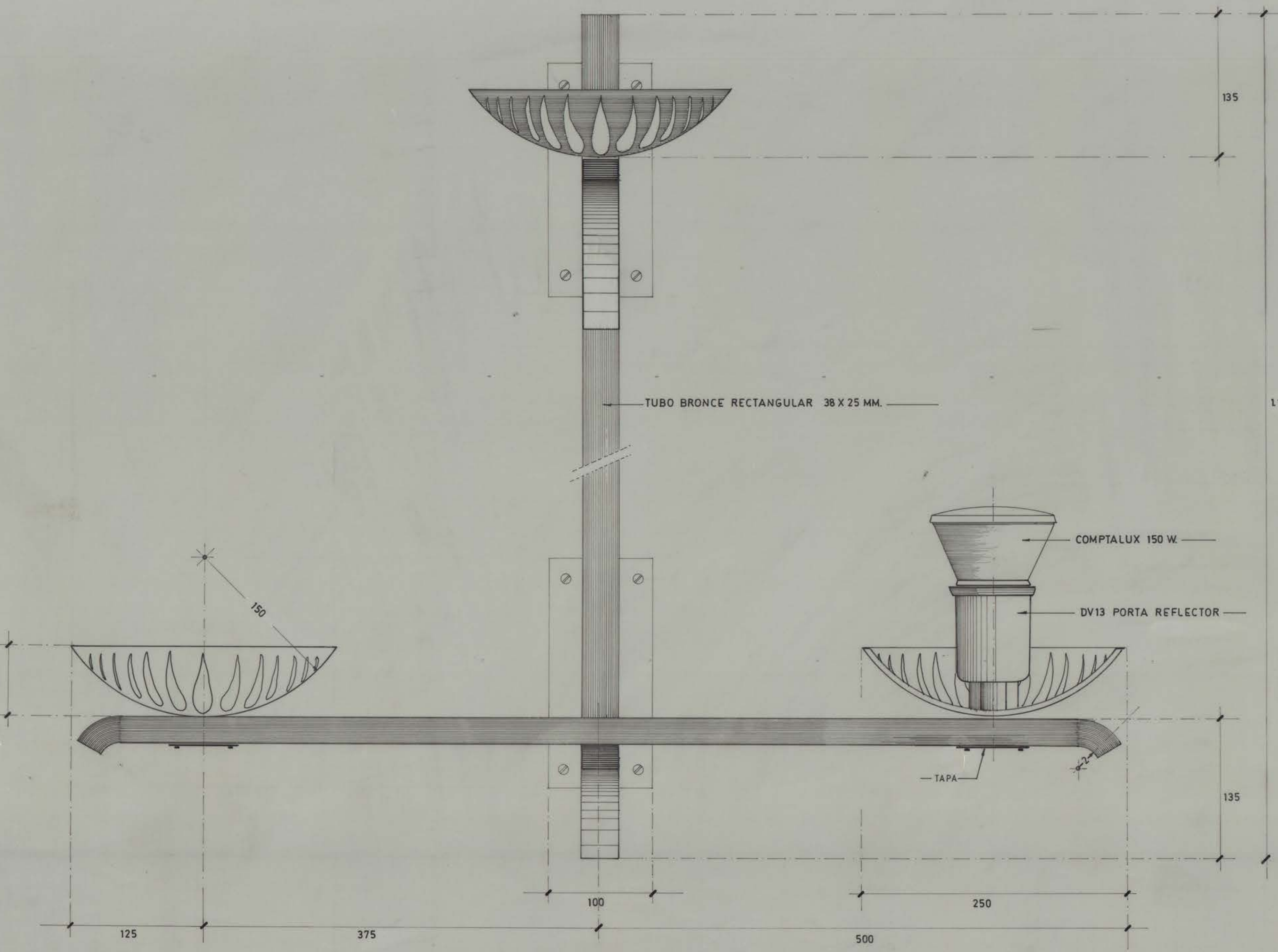
ELEVACION FRONTAL ESC. 1:2,5
