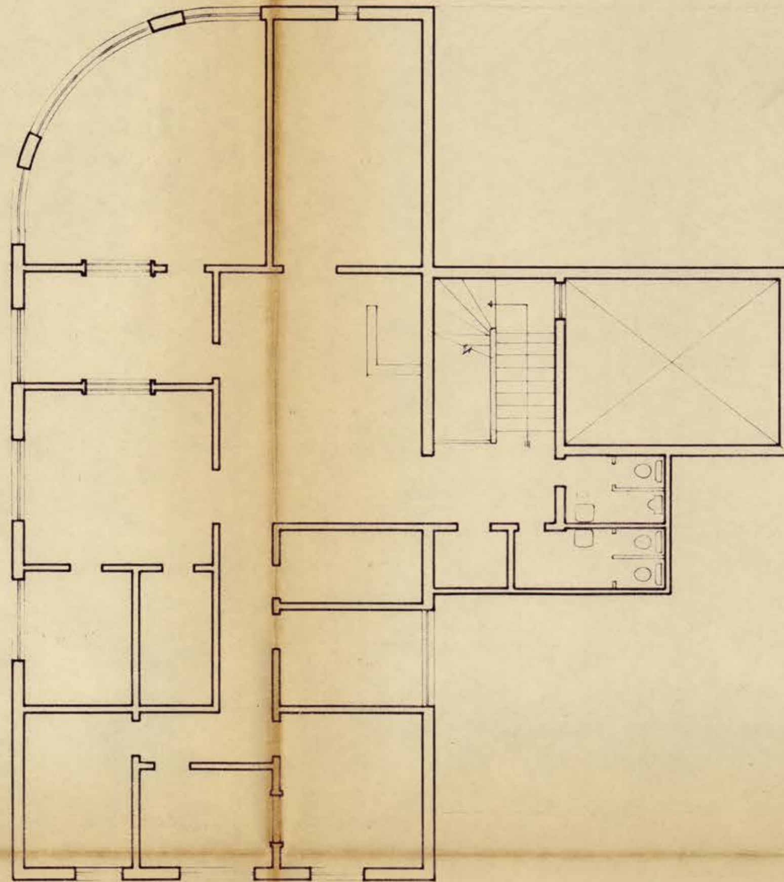
PLANTA 4° piso Inst. Quím. y Farmacia Esc. 1 : 100
