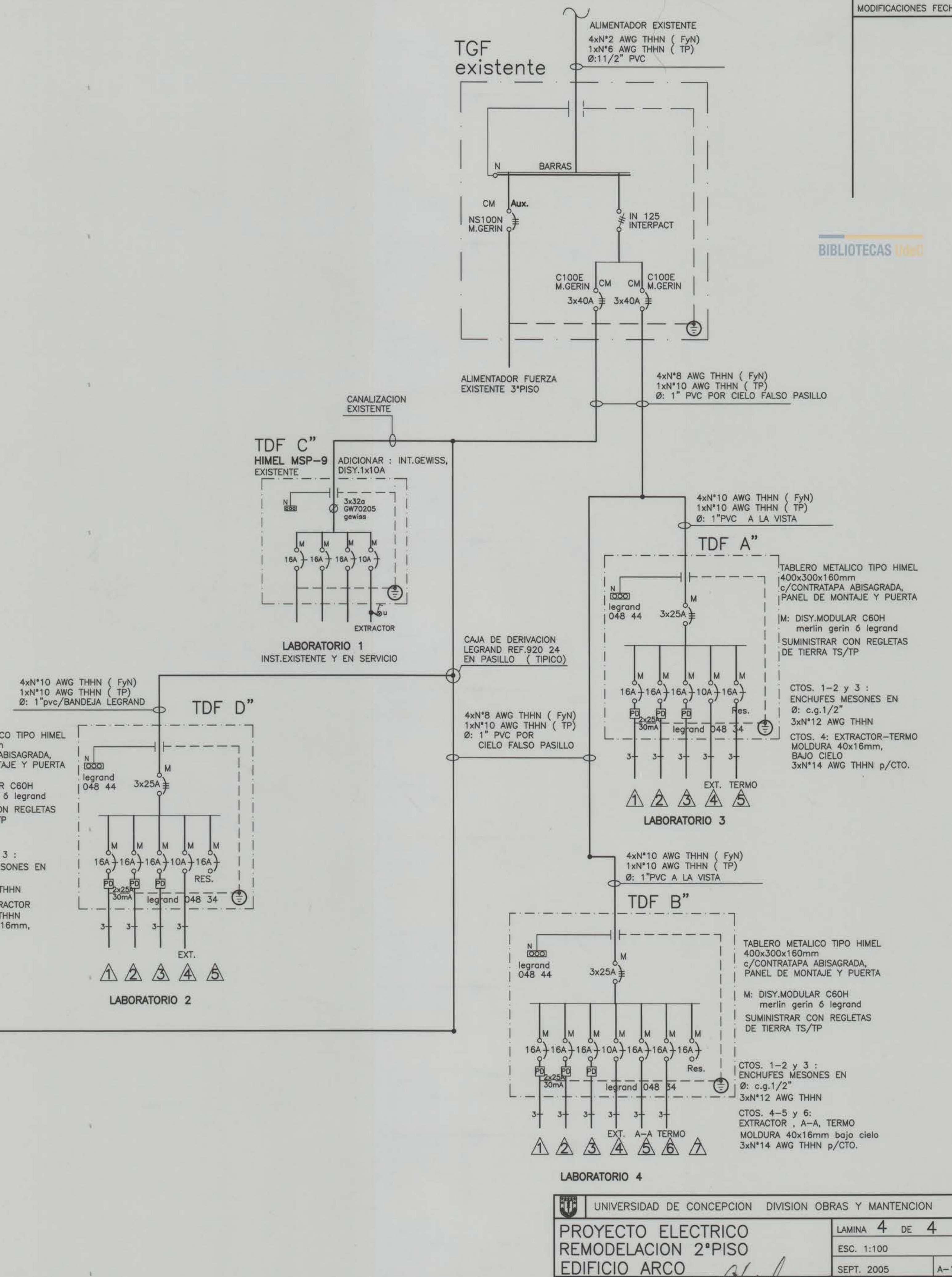
DIAGRAMA UNILINEAL FUERZA
