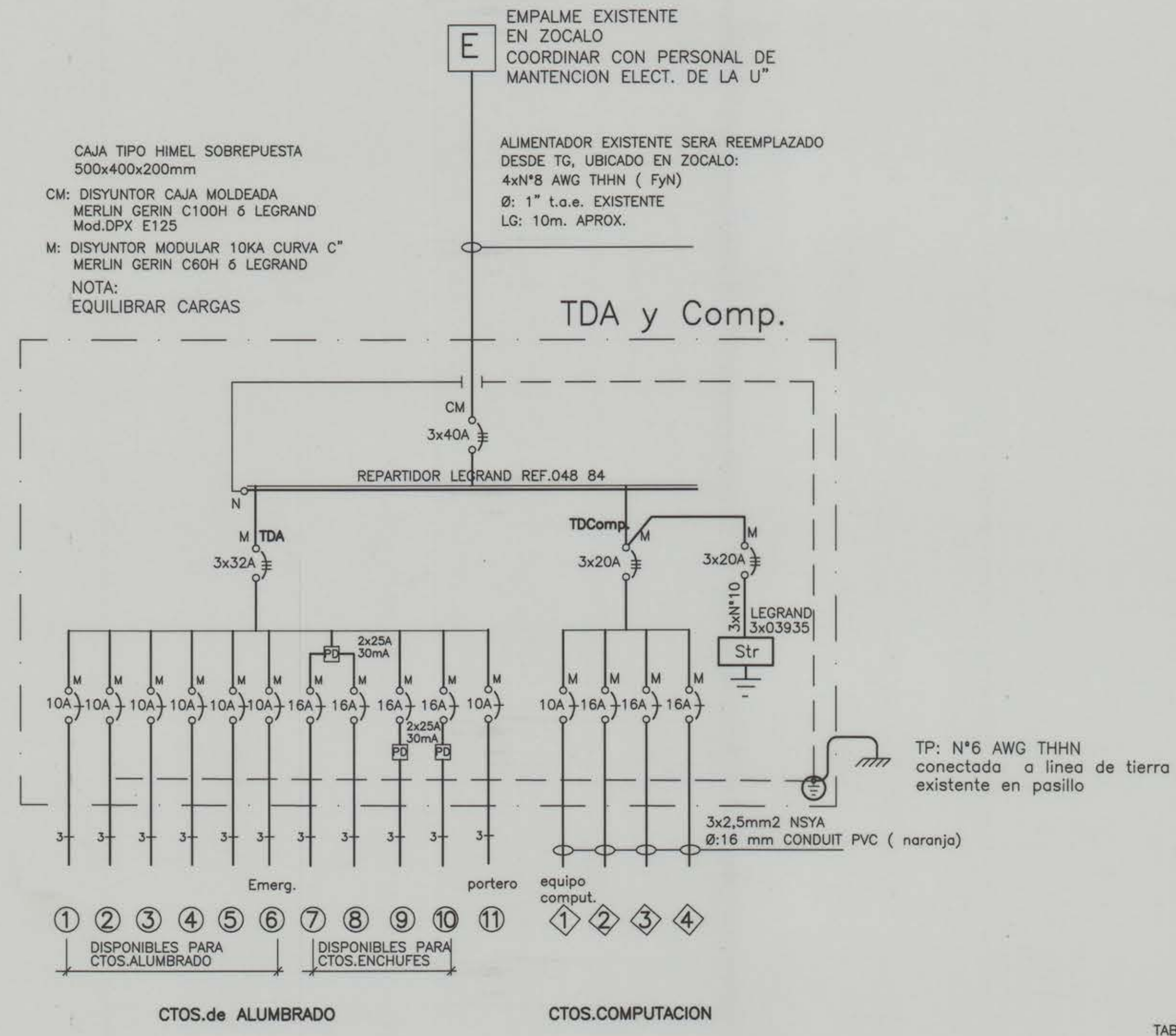
DIAGRAMA UNILINEAL ALUMBRADO Y COMPUTACION
