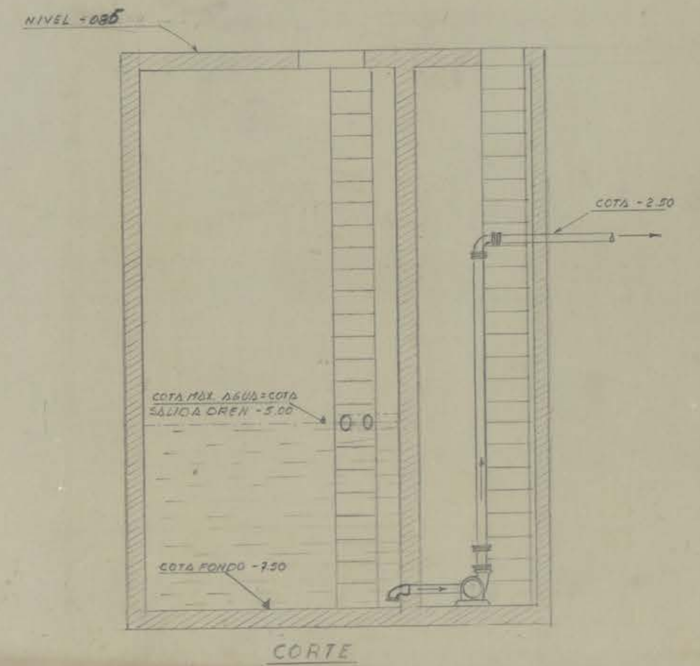
DETALLE ESTANQUE DE ACUMULACION ESCALA 1:50
