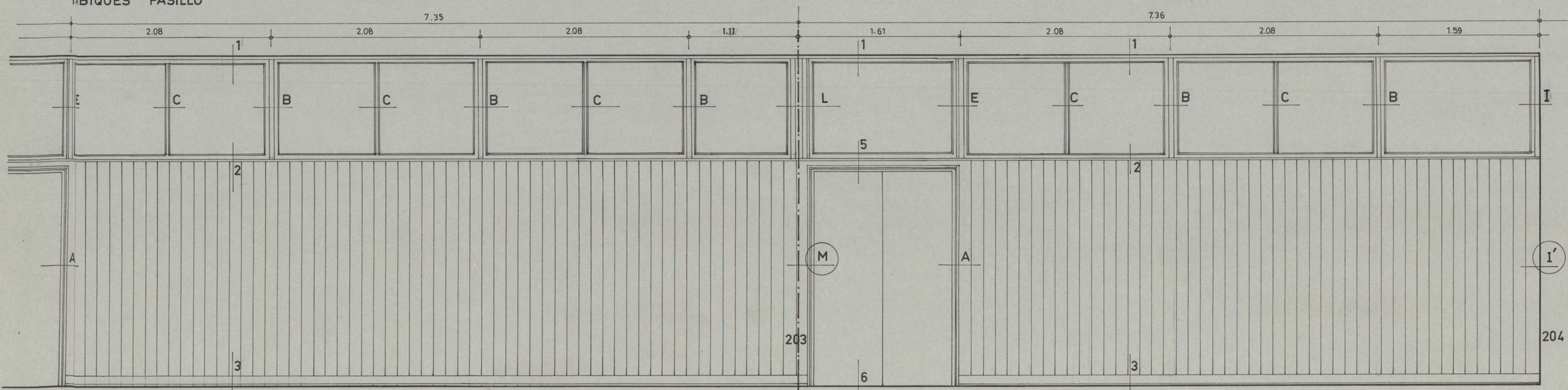
TABIQUES PASILLO
