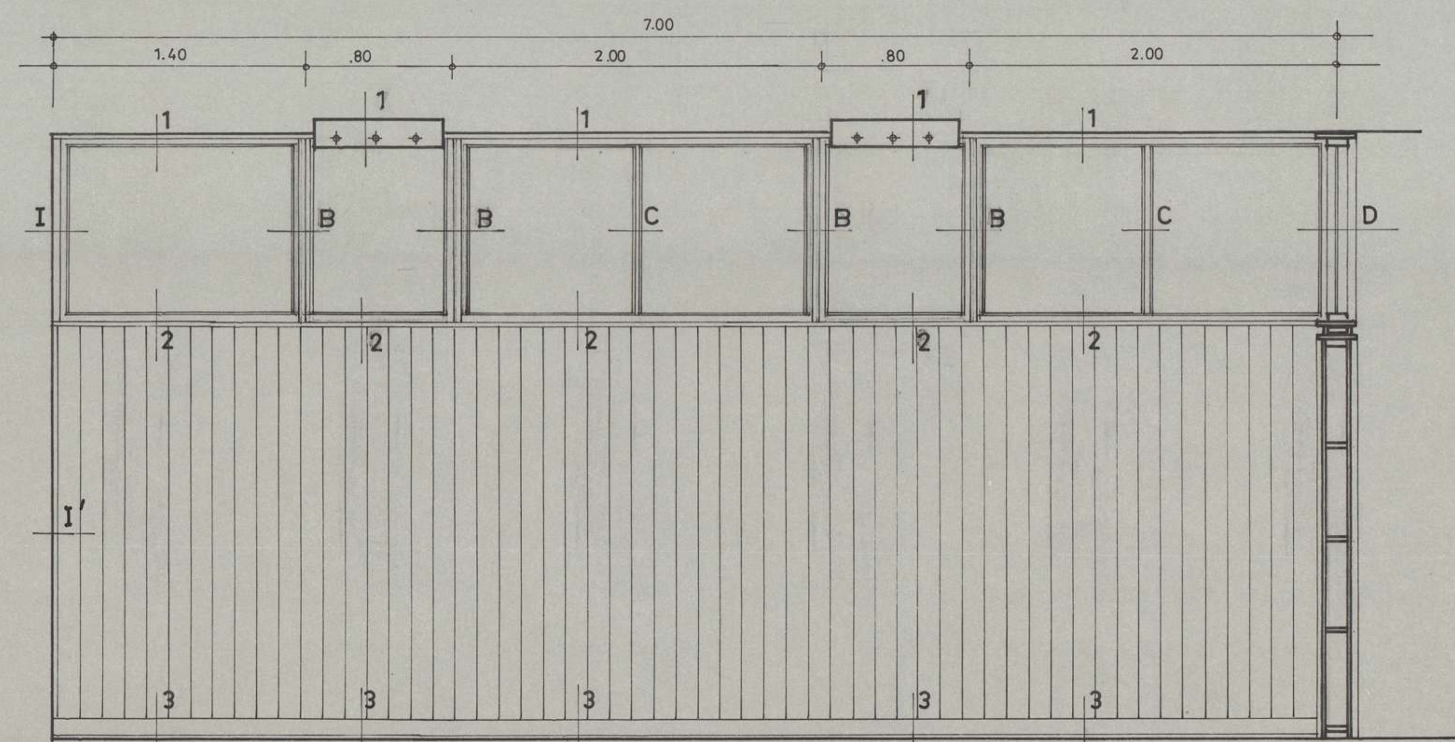
TABIQUES ENTRE SALAS (TRES PAÑOS IGUALES)
